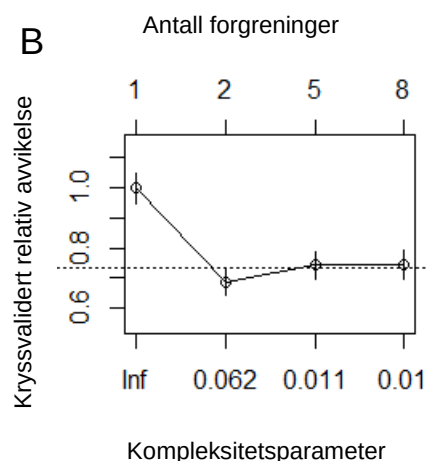
Figur 10. A) Klassifikasjonstre til analyse av sannsynligheten for at en karplante er forvillet, samt hvilke egenskaper som karakteriserer arter som kommer inn via denne spredningsveien. B) Kryssvalidering til utvalgelse av den optimale størrelse på treet. Se figur 9B for forklaring.
