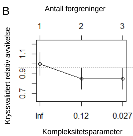
Figur 9. A) Klassifikasjonstre til analyse av sannsynligheten for at en karplante har etablert seg i Norge som følge av direkte utsetting i naturen, samt hvilke egenskaper som karakteriserer arter som kommer inn via denne spredningsveien. B) Kryssvalidering til utvelgelse av den optimale størrelse på treet. Det optimale treet er det med det minste antall forgreninger, der den kryssvaliderte relative avvikelse ligger innenfor \pm 1 standardavvikelse fra minimum. Den stiplede linjen angir den øvre grensen av denne standardavvikelsen, og det beste tre er dermed det første som ligger under denne linjen.
