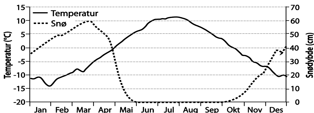
Figur 11. Lufttemperatur og akkumulert snømengde i Abisko, Sverige, for januar til desember, beregnet for normalperioden 1961-1990. Kilde: Abisko naturvetenskapliga station ( www.polar.se ).
