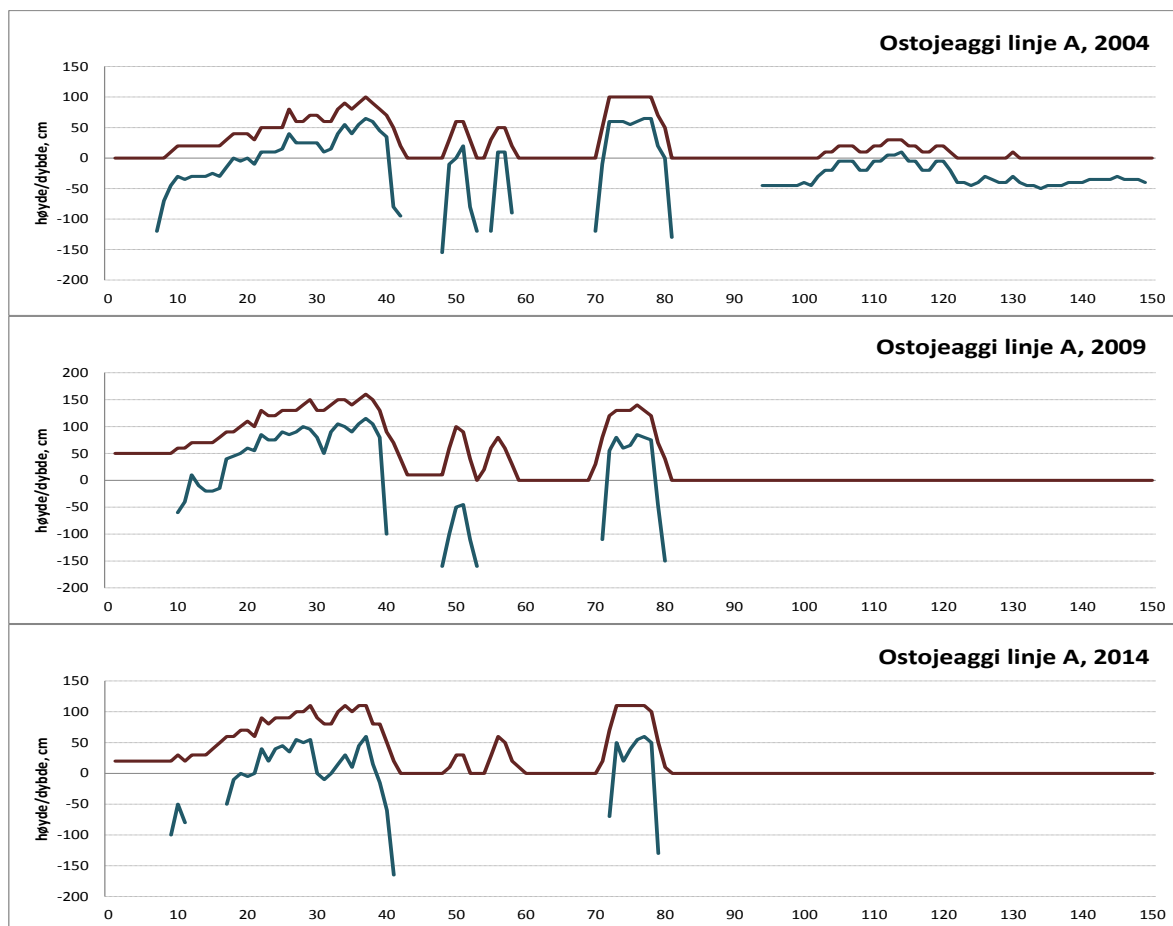
Figur 21. Høydestruktur og teledybde for linje A i 2004, 2009 og 2014. Brune linjer viser mark-høyde og blå linjer teleforekomstens dybdenivå under overflaten. Merk at høydenivå ble målt noe forskjellig i de tre årene (grunnet myrass hellings). © NINA 2015.
