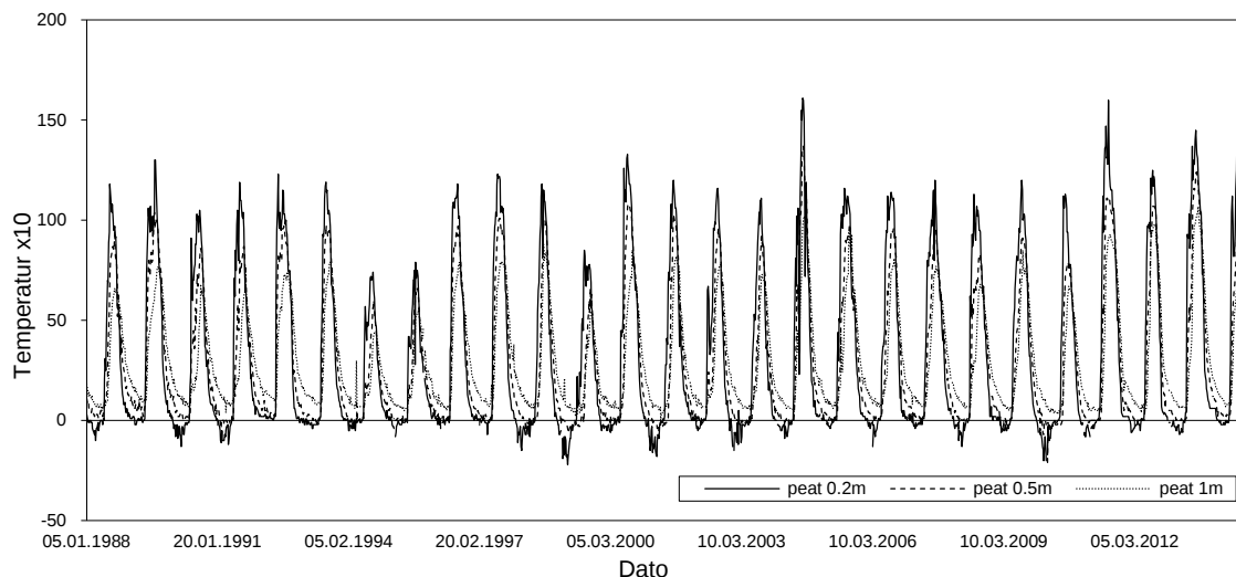
Figur 8. Temperaturutvikling på tre ulike jorddybder (0,2 m, 0,5 m og 1 m) i torvmark i Abisko, Sverige, 1988-2014. Kilde: Abisko naturvetenskapliga station ( www.polar.se ). © NINA 2015.
