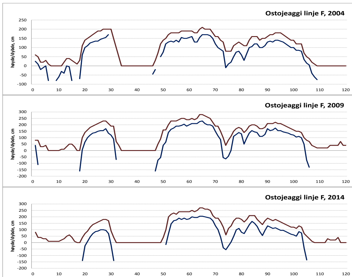
Figur 23. Høydestruktur og teledybde for linje F i 2004, 2009 og 2014. Brune linjer viser markhøyde og blå linjer teleforekomstens dybdenivå under overflaten. Merk at maksimalt høydenivå ble målt noe forskjellig i de tre årene (grunnet myras helling). © NINA 2015.
