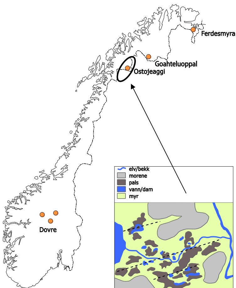
Figur 4. Studiedesign med utvalgte overvåkingsområder i Sør- og Nord-Norge. Området som er presentert i denne rapporten, er markert med en oval. Det innfelte kartet viser eksempel på palsområde med analyselinjer for innsamling av abiotisk og biotisk datamateriale. © NINA 2015.
