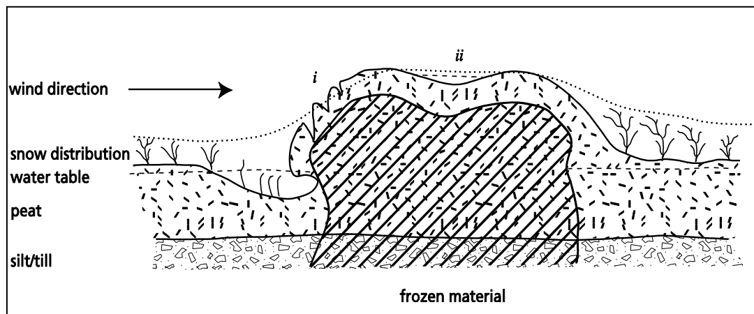
Figur V2. Palsuppbyggnad, grundvattennivå i omgivande myrmark, och snöns fördelning under högvintern. Palsens frusna kärna är omgiven av ofrusen torv under sommaren, och vegetationens struktur på och runt palsen är formad av vind och snöförhållanden under vintern. i) exponerad yta som utsätts för vind och erosion; ii) tillfällig vattensamling (källa: Hofgaard 2003). © NINA 2015.
