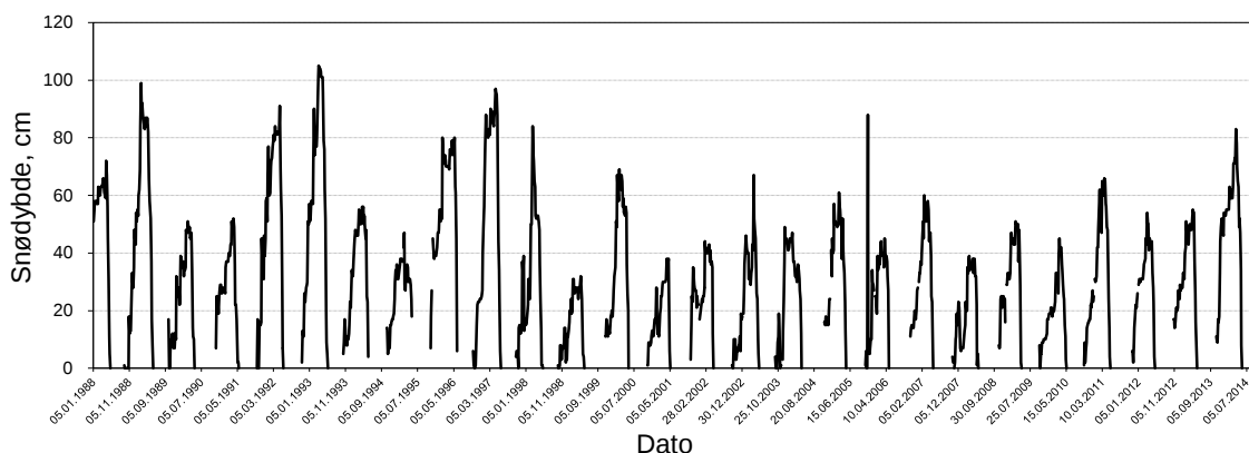
Figur 10. Snødybde fra målestasjonen i Abisko, Sverige, for perioden 1988 til 2014. Kilde: Abisko naturvetenskapliga station ( www.polar.se ). © NINA 2015.
