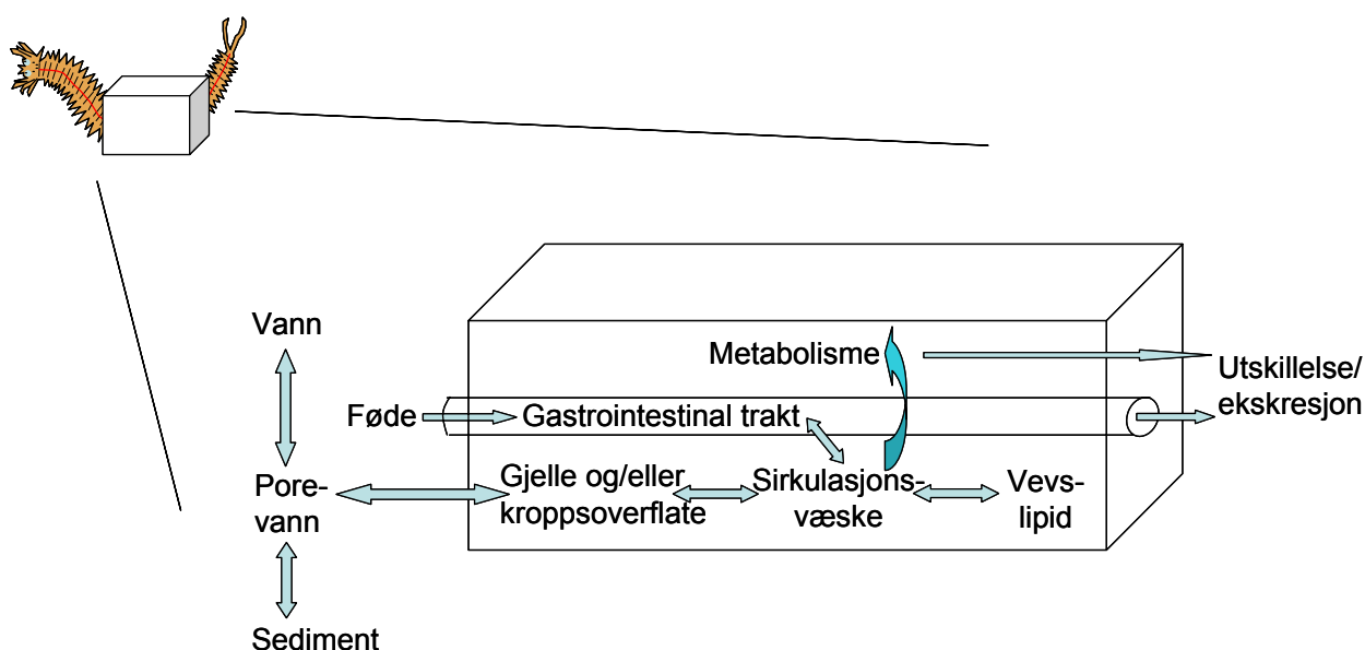
Figur 2. Skjematisk fremstilling av veier og mekanismer som teoretisk er involvert i bioakkumulering av PAH i benthiske organismer. Det innstilles en likevekt mellom partikkelbundet PAH og PAH løst i porevannet mellom sedimentpartiklene. Likeledes innstilles det en likevekt mellom PAH i porevann og vannet over sedimentet. Det innstilles også en likevekt mellom løst PAH og fettfaser i organismen (via sirkulasjonssystemet). For infauna (organismer som lever i sedimentet) skjer diffusjonen over kroppsoverflate og særlig respirasjonsoverflater, men også over tarmveggen for de organismene som inntar (spiser) sediment. Forhold i tarmen kan også føre til økt desorpsjon (og biotilgjengelighet) for PAH og andre forbindelser, som omtalt i teksten (nedenfor). Enkelte organismer har evne til å omdanne ('biotransformere'/metabolisere) enkelte forbindelser og skille ut mer vannløselige omdannelsesprodukter ('metabolitter'). Andre mekanismer som kan være involvert i bioakkumulering i akvatiske organismer (ikke vist her) er 'vekstfortynning' (lavere konsentrasjon som følge av at volumet av organismen øker) og eventuell utskillelse av fremmedstoffer gjennom at organismen slipper gytteprodukter.
